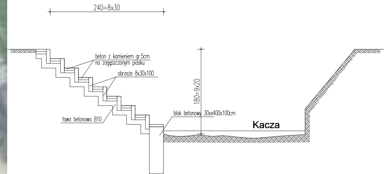
schody 9x 20x 30
